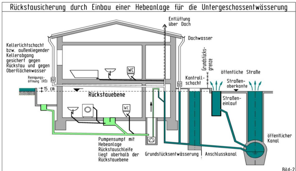
Bild 2: Rückstausicherung durch Hebeanlage
