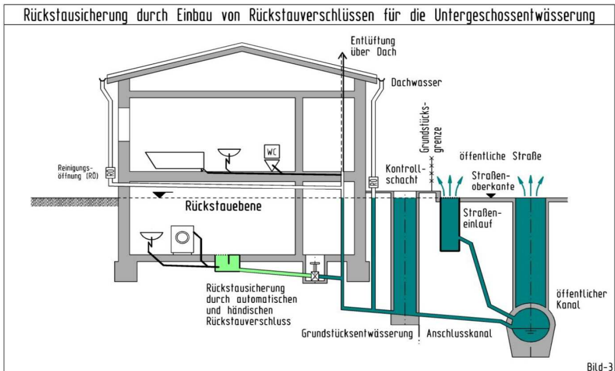
Bild 3: Rückstausicherung durch Rückstauverschluss
