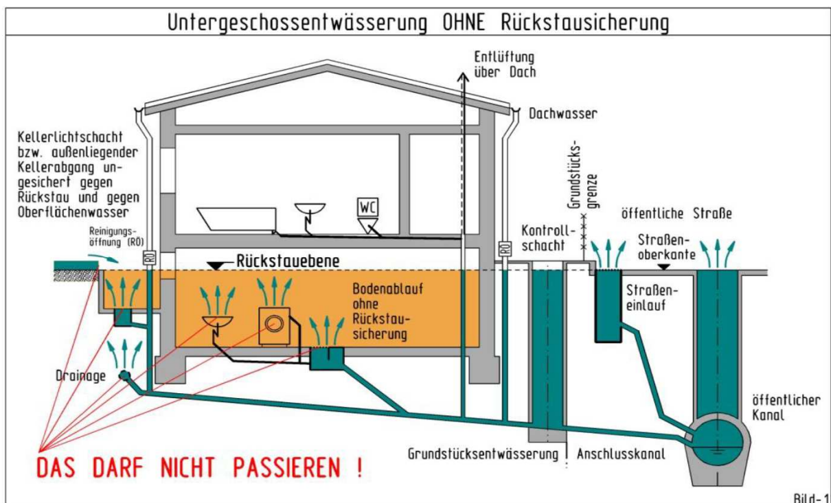
Bild 1: Entwässerung Untergeschoss ohne Rückstausicherung
